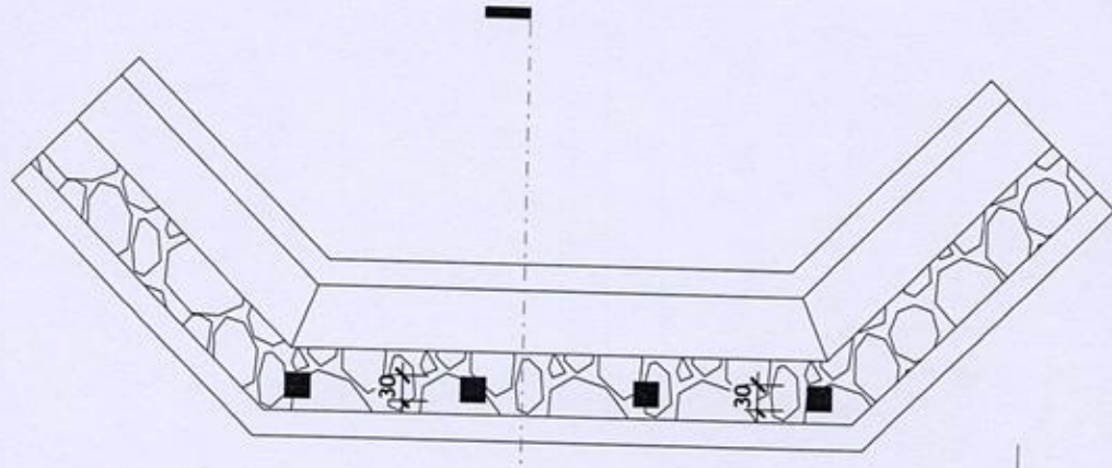
1 Column/Pillar Plan Ech : 1 : 60
