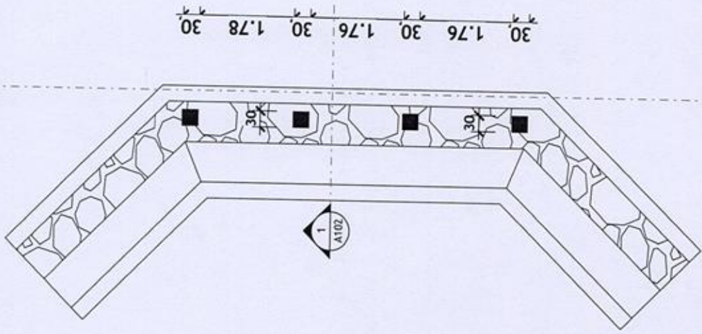
1 Column/Pillar Plan Ech : 1 : 60
